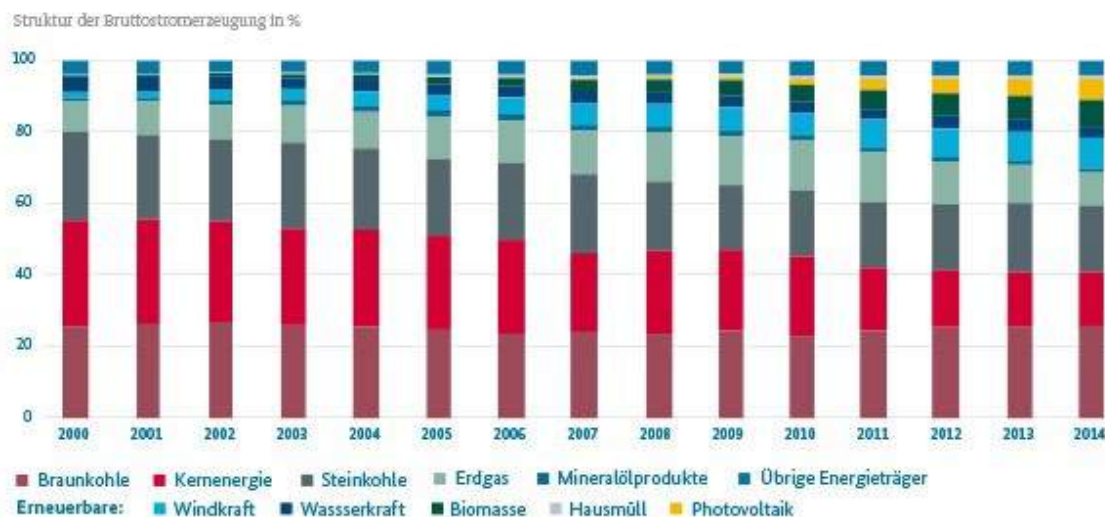
Graf 26 – Skladba výroby elektrické energie podle zdroje v Německu, 2014.
