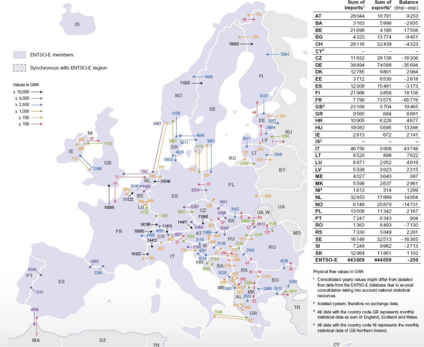
Příloha 9 - Fyzické toky elektřiny mezi státy Evropy v r. 2014
