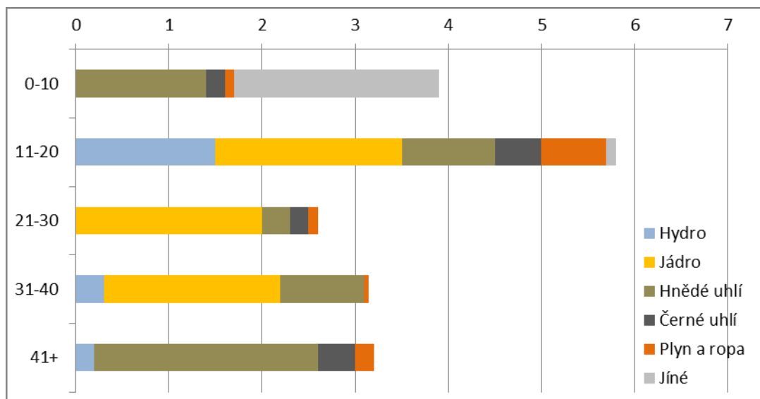
Stáří zdrojů dle druhů paliv v GW (2011)
