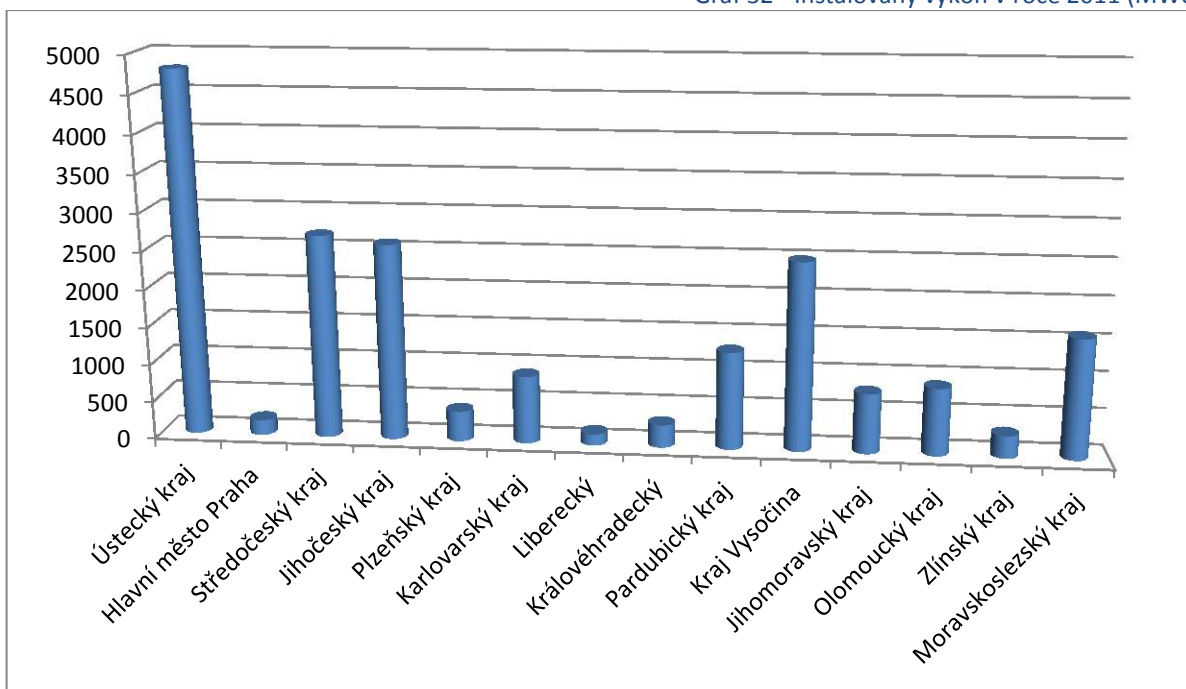
Graf 32 - Instalovaný výkon v roce 2011 (MWe)
